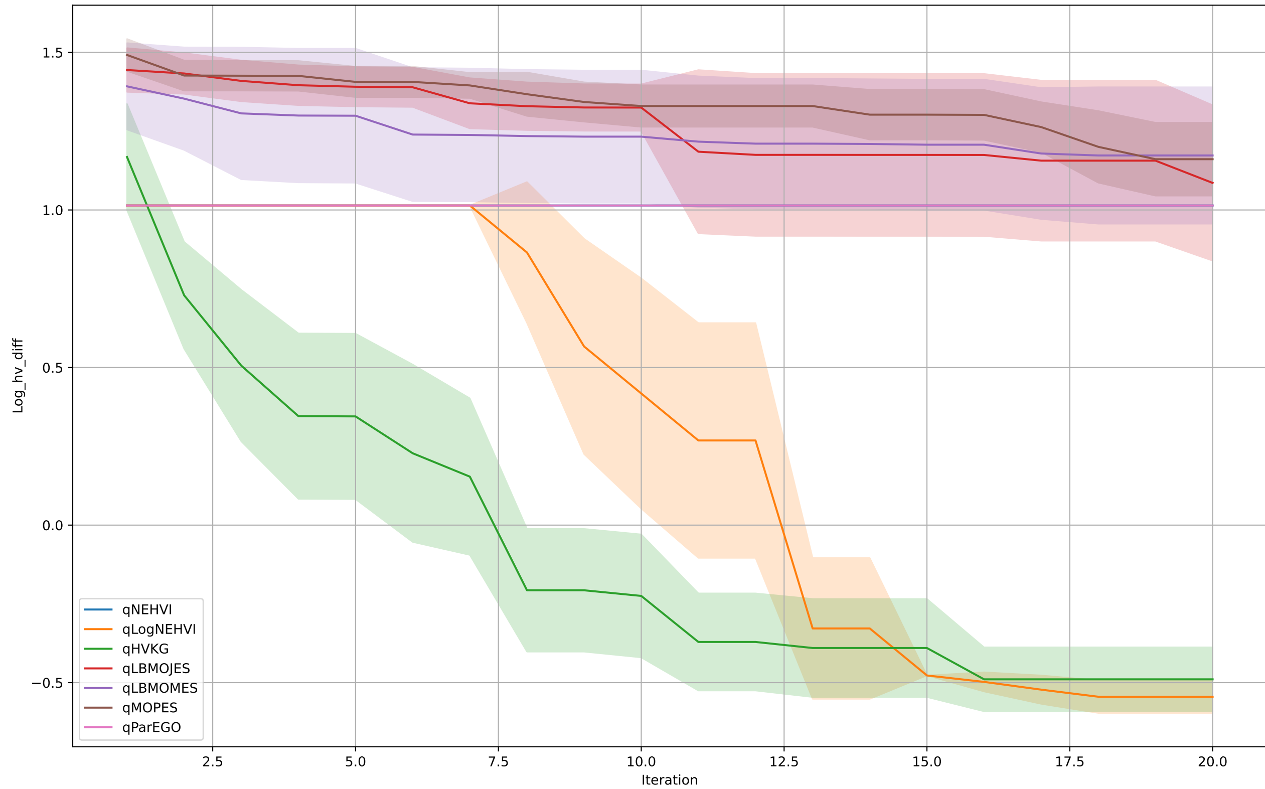
ZDT2
