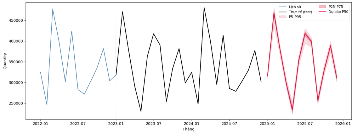
Hình 4.9: Fan chart toàn bộ: 3 năm lịch sử gần nhất, tập test 2023-2024 (thực tế), và dự báo phân vị 12 tháng tới (2025). Vùng đỏ đậm: P25-P75; vùng đỏ nhạt: P5-P95.
