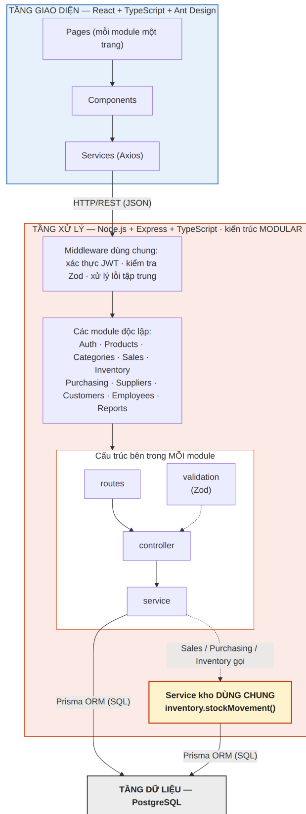
Hình 3.1: Kiến trúc ba tầng kết hợp tổ chức modular ở backend
