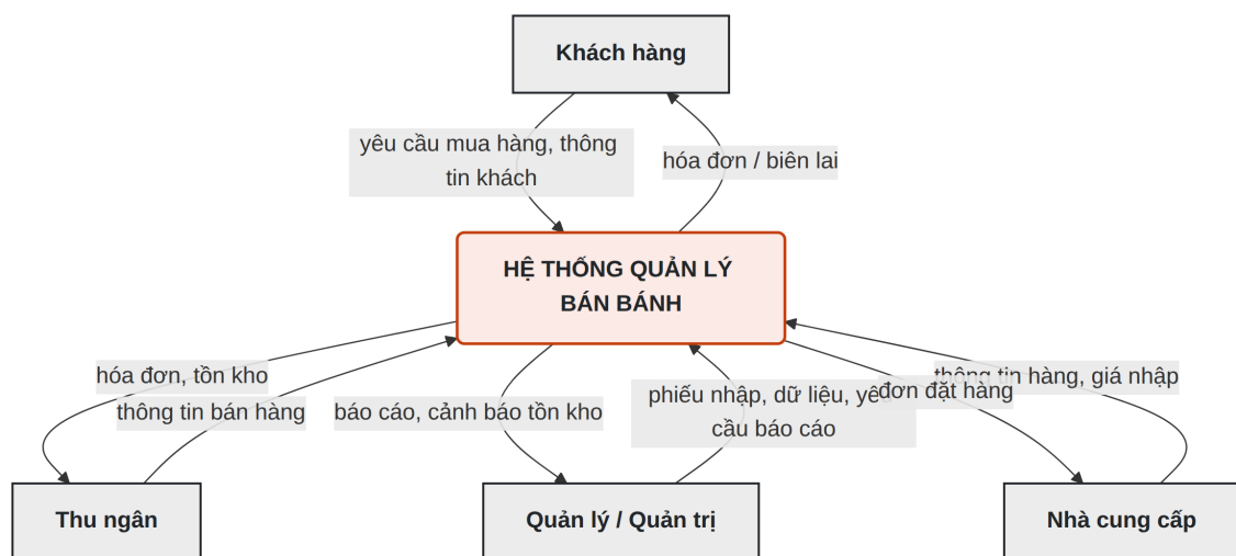
Hình 2.3: Biểu đồ luồng dữ liệu mức ngữ cảnh
