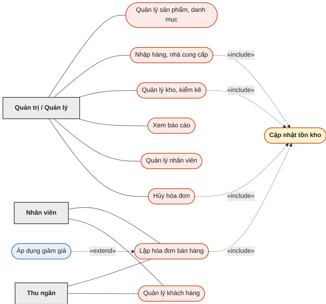
Hình 2.2: Biểu đồ use case tổng quát
