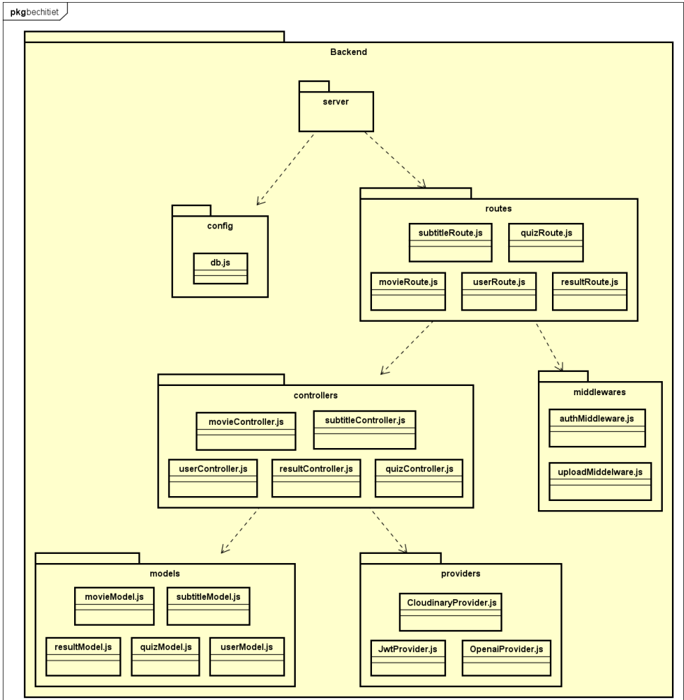
Sơ đồ gói chi tiết phía Backend
