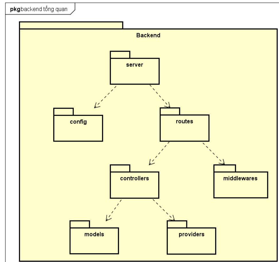
Sơ đồ gói tổng quan phía Backend
