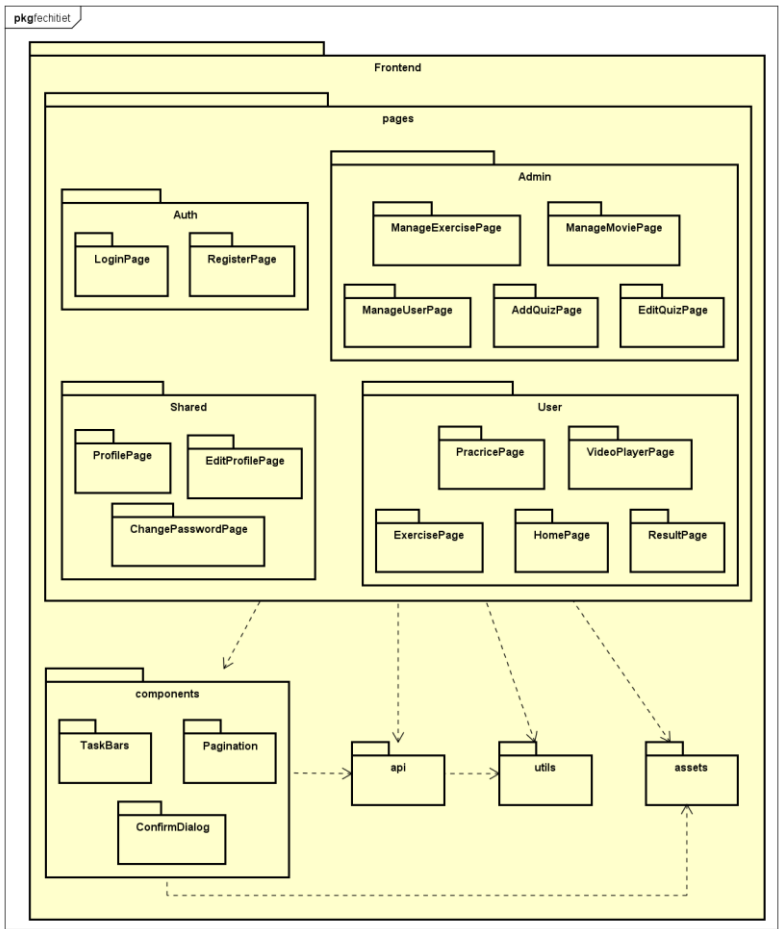
Sơ đồ gói chi tiết phía Frontend
