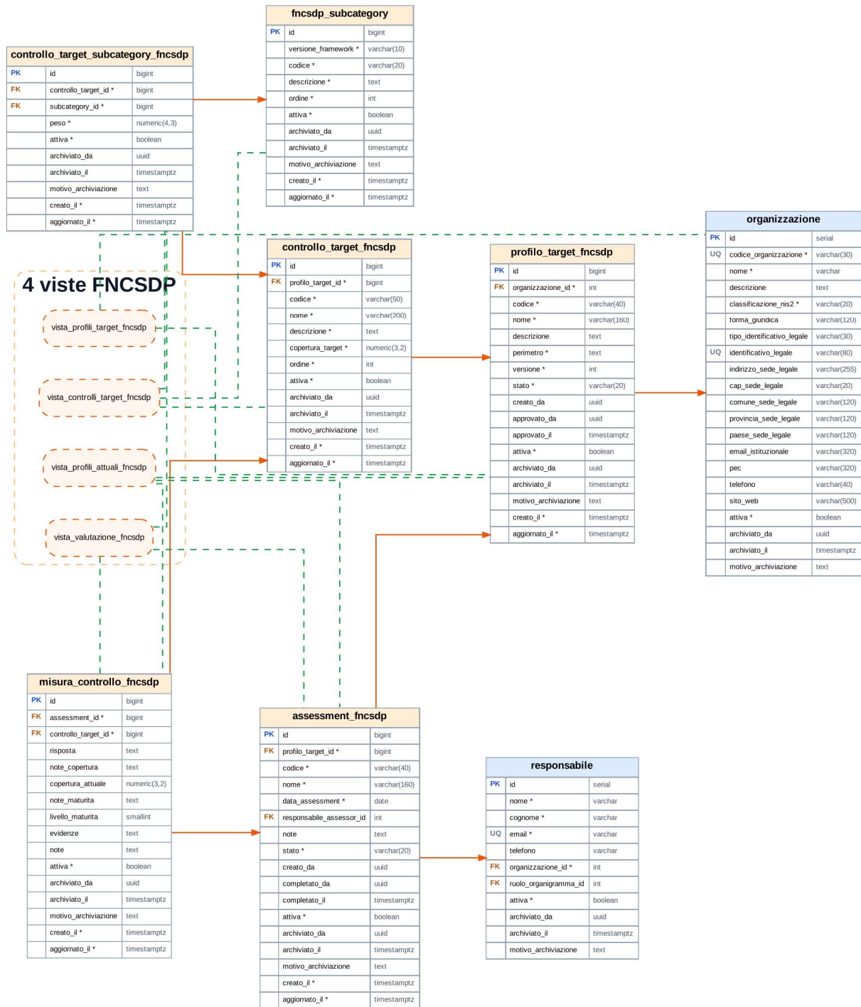
Figura 3 — Dettaglio ER del modulo Assessment FNCSDP: sei tabelle normalizzate, quattro viste e collegamenti al soggetto NIS2 e all'assessor.
