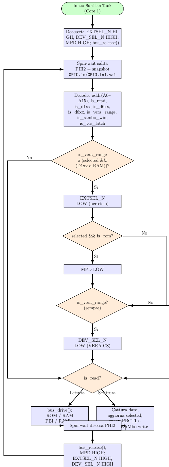
Figura 2: Diagramma di flusso semplificato del MonitorTask (modalità PBI, ESP32-S3FN8).
