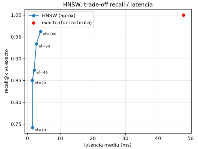
Figura 5. HNSW: curva recall-latencia al variar ef_search.
