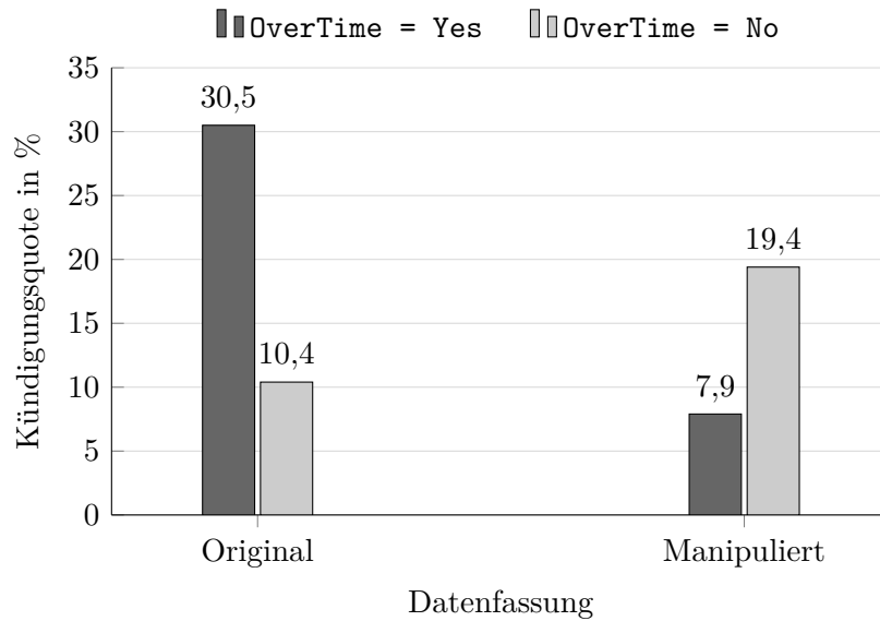
Abbildung 3.2: Kündigungsquoten nach OverTime im ursprünglichen und manipulierten Datensatz. Die Randverteilungen bleiben in beiden Fassungen identisch, mit 416 Beschäftigten mit und 1054 ohne Überstunden sowie unveränderter Gesamtkündigungsquote; umgekehrt wird allein die Richtung des Zusammenhangs zwischen beiden Variablen.
