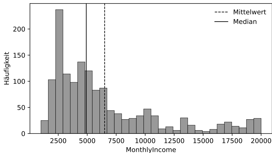
Abbildung 2.2: Verteilung der Variable MonthlyIncome im verwendeten Datensatz. Der Mittelwert liegt rechts vom Median, was für eine rechtsschiefe Verteilung charakteristisch ist.
