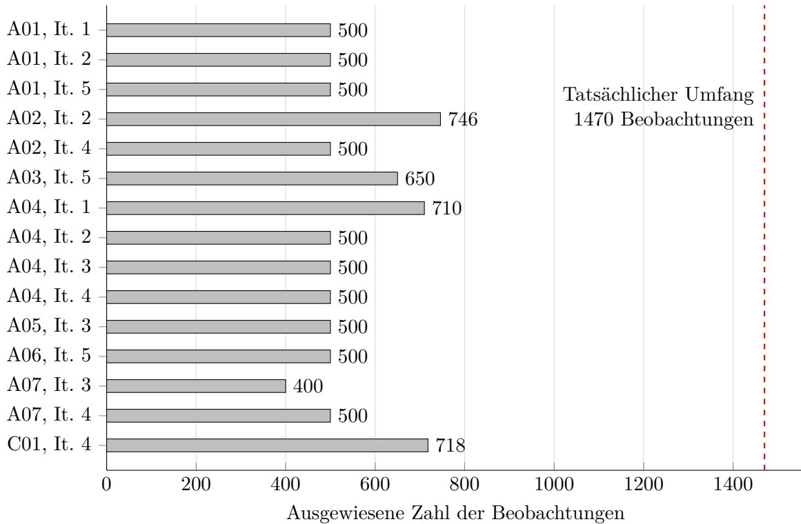
Abbildung 4.2: Von Gemini ausgewiesene Beobachtungszahlen im Vergleich zur tatsächlichen Größe des übergebenen Datensatzes. Aufgeführt sind alle Antworten, in denen der Umfang der zugrunde gelegten Datengrundlage ausdrücklich genannt wird, jeweils mit Frage und Iteration.
