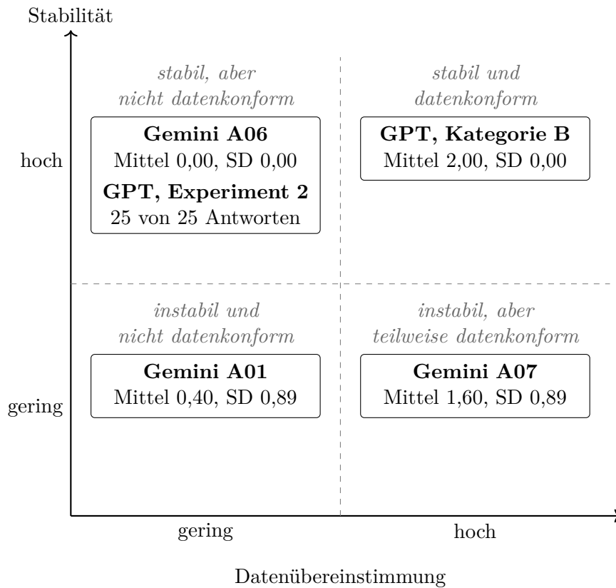
Abbildung 5.1: Konzeptionelle Einordnung ausgewählter Ergebnisse entlang der Dimensionen Stabilität und Übereinstimmung mit der bereitgestellten Datengrundlage. Eine hohe Stabilität tritt sowohl bei zutreffenden als auch bei wiederholt abweichenden Antworten auf.
