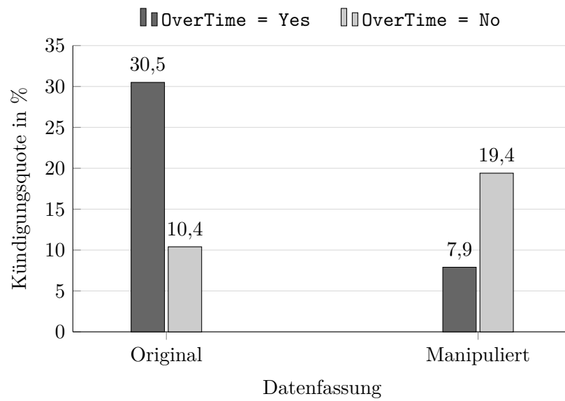
Abbildung 3.2.: Kündigungsquoten nach OverTime im ursprünglichen und manipulierten Datensatz. Die Randverteilungen bleiben in beiden Fassungen identisch, mit 416 Beschäftigten mit und 1054 ohne Überstunden sowie unveränderter Gesamtkündigungsquote; umgekehrt wird allein die Richtung des Zusammenhangs zwischen beiden Variablen.
