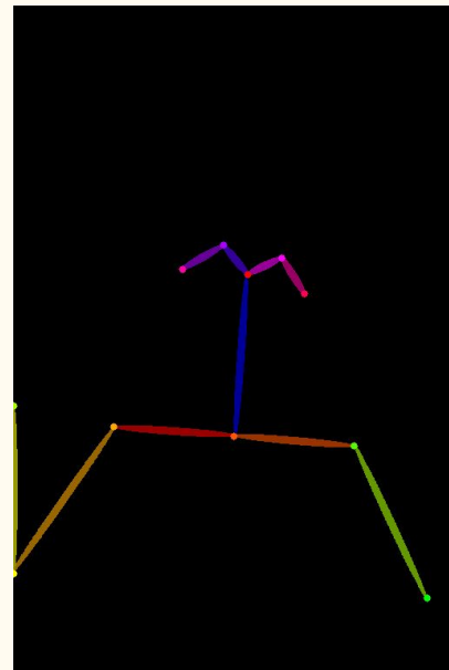
Ảnh Keypoint
