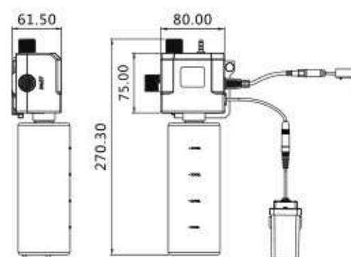
感应皂液二合一控制盒组件
