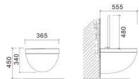
挂式座便器 G13305 ¥2258
