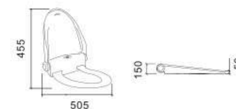
自动便洁垫 G31520 ¥2620
