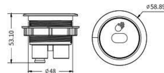
挥手感应水件总成 BC-31515 ¥520
