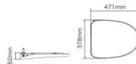
恒温加热盖板 GBL-1186A ¥672
