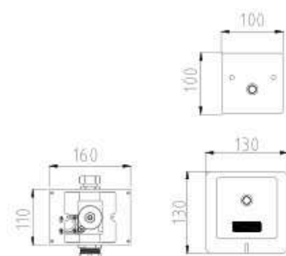
感应蹲便冲水器 GBL-8300M2Li ¥2360 GBL-8300M2/AD ¥2380
