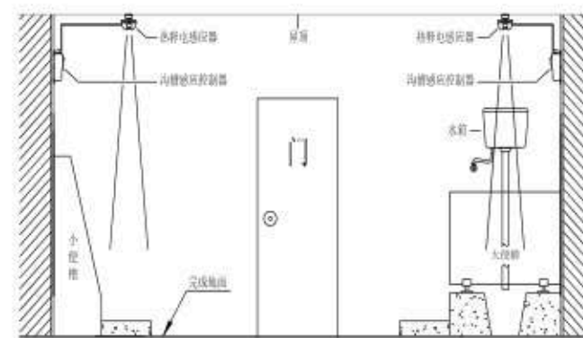
安装图 GBL-6710A安装示意图。
