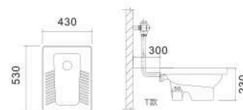
蹲便器 G13105T ¥458 G13105F ¥428
