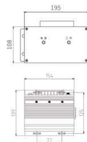
安装图 GBL-6710A安装示意图。
