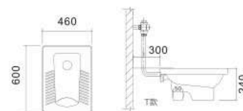
蹲便器 G13113T ¥740 G13113F ¥686
