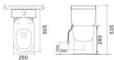
儿童座便器 G13216 ¥1280
