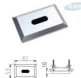
感应小便冲水器 GBL-6231D1 ¥705 GBL-6231D2 ¥605
