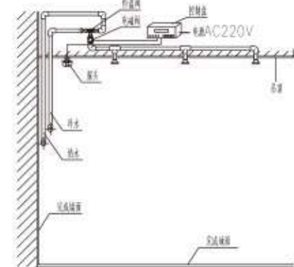
安装图 GBL-6416安装示意图
