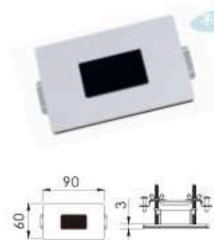
感应小便冲水器 GBL-6236D1 ¥650 GBL-6236D2 ¥550
