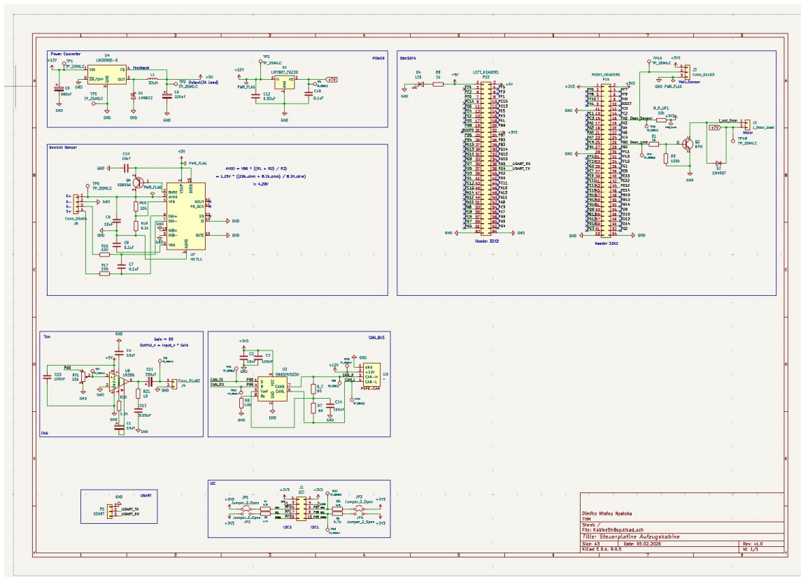
Abbildung 1: Vollständiger Schaltplan der entwickelten Leiterplatte
