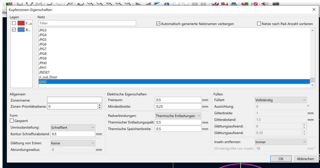
Abbildung 6: Konfiguration der GND-Kupferzone: vollständige Füllung, thermische Entlastungen
