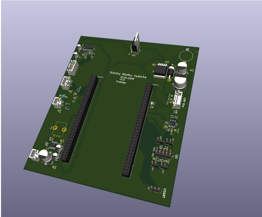
Abbildung 8: 3D-Darstellung der bestückten Leiterplatte
