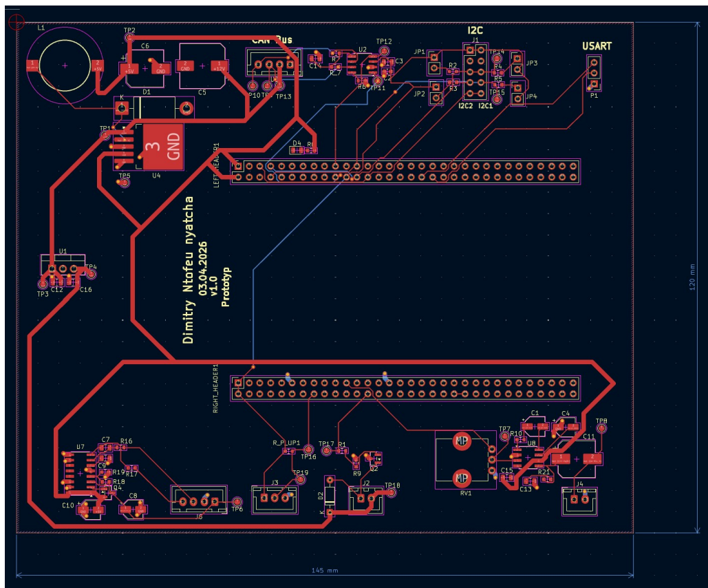
Abbildung 7: PCB-Layout der Leiterplatte (KiCad)
