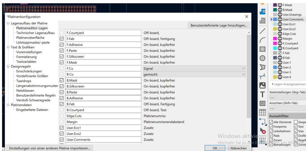
Abbildung 4: Lagenkonfiguration der Leiterplatte in KiCad: F.Cu als Signallage, B.Cu als gemischte Lage (Massefläche)
