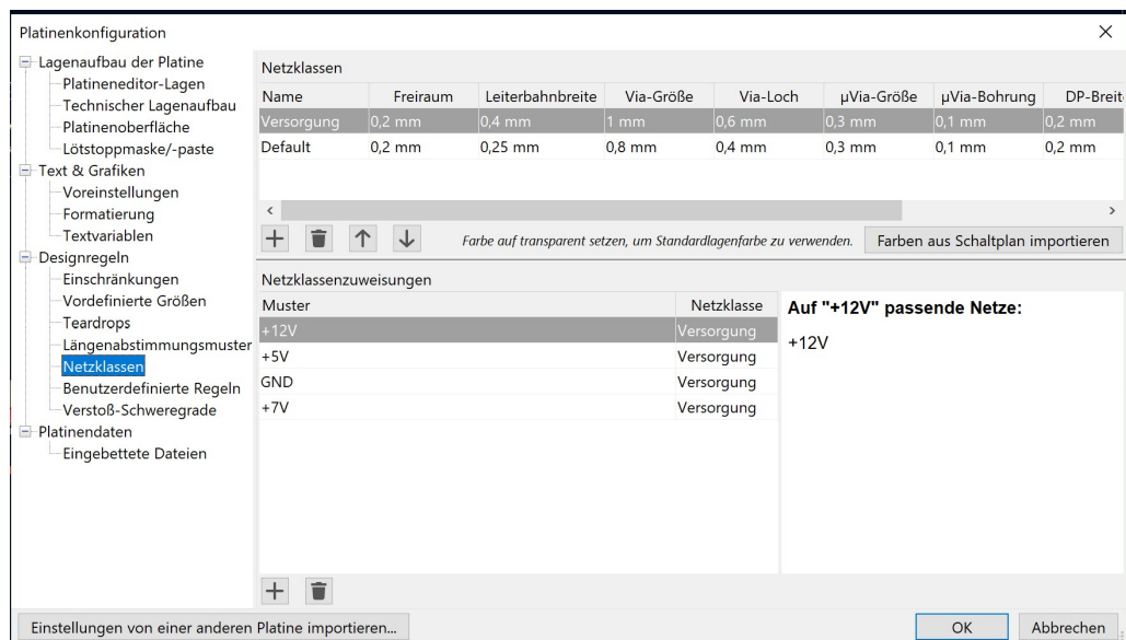
Abbildung 5: Definition der Netzklassen in KiCad mit den zugehörigen Designregeln für Versorgungsnetze und Signalnetze
