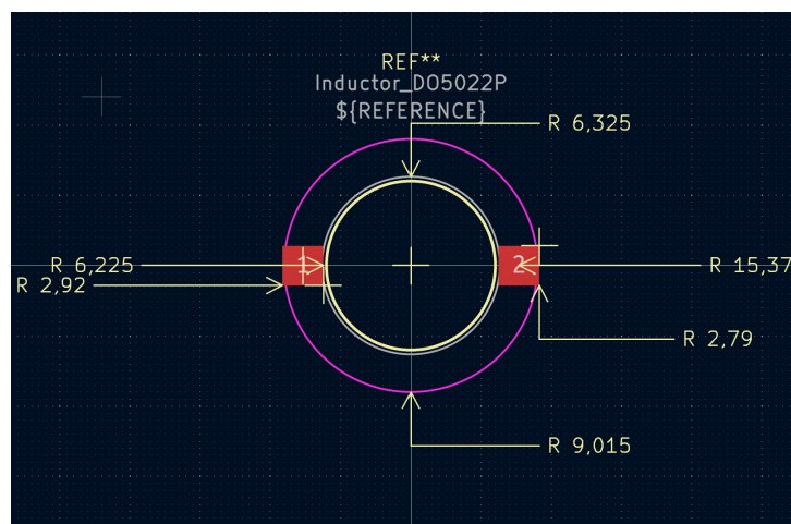
Abbildung 2: Erstellter PCB-Footprint der Induktivität DO5022P-333. Die Abmessungen basieren auf dem Recommended Land Pattern der Hersteller-Datasheet (vgl. Anhang, Datasheet DO5022P).
