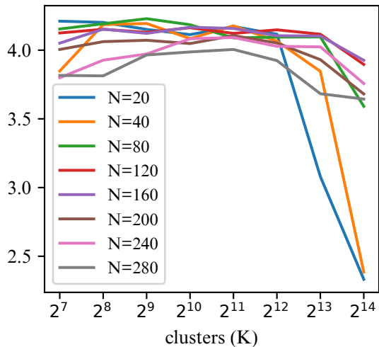
UTMOS
