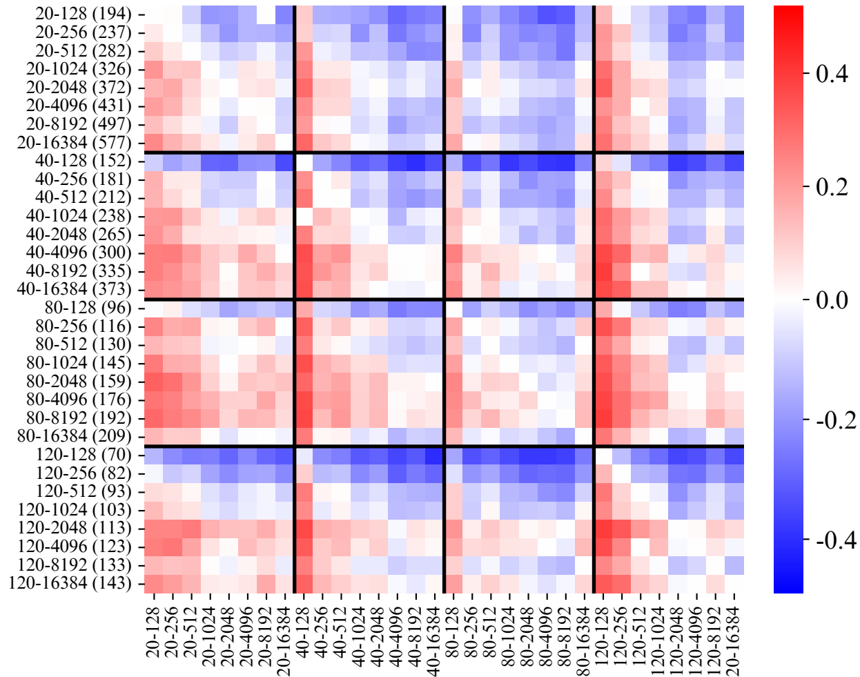
VITS
