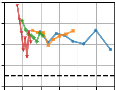
VITS
