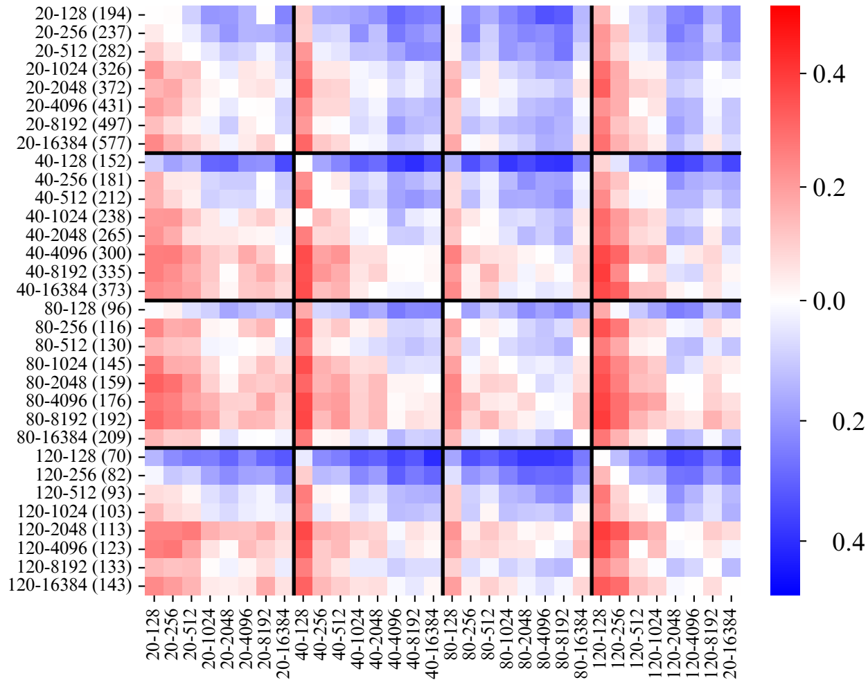
VITS
