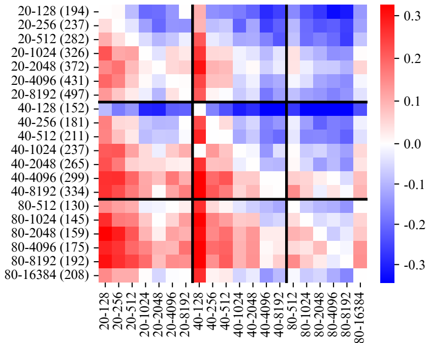
vits
