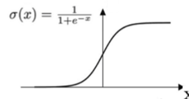
Sigmoid Function
