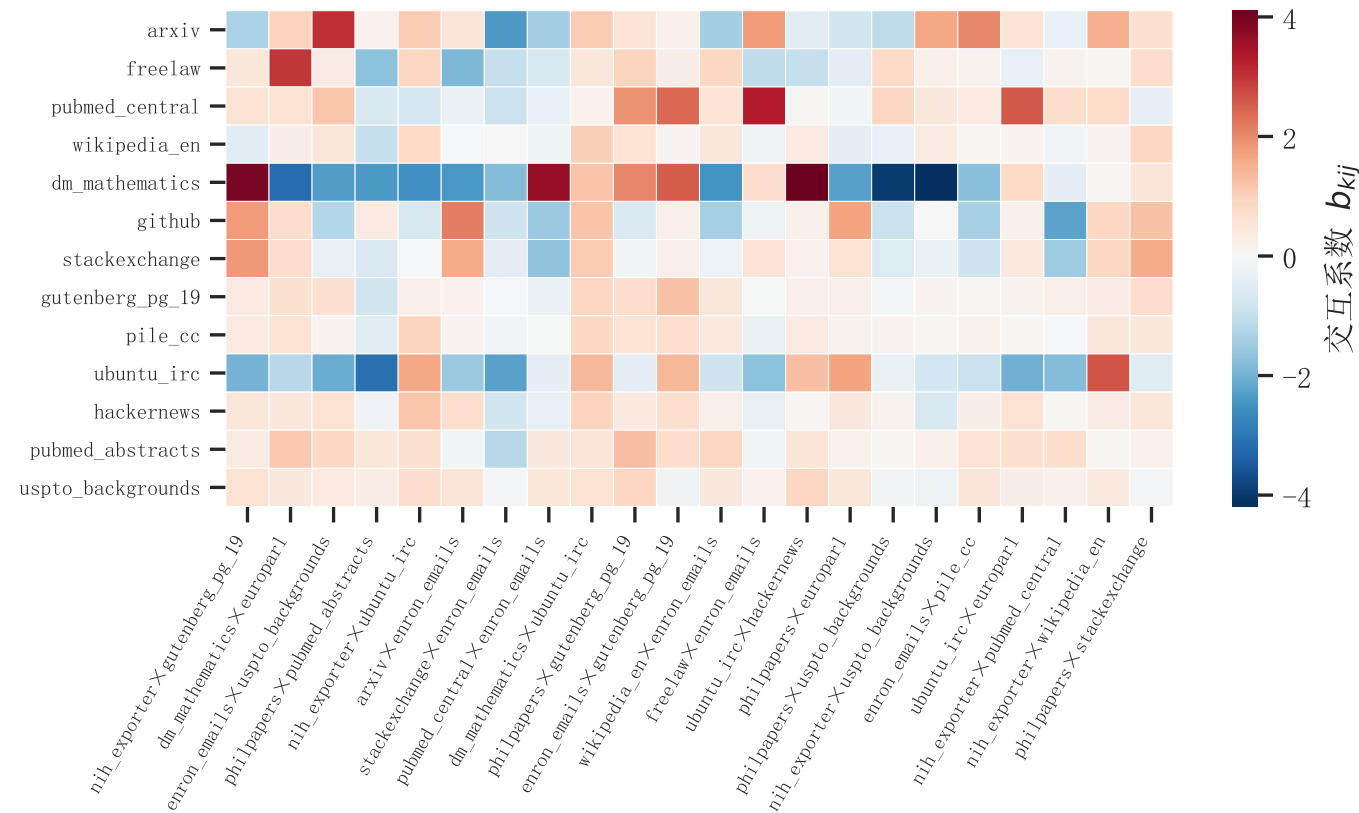
(a) 交互项系数 (按平均绝对强度取前 22)
