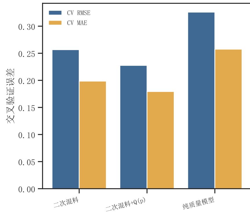
配比模型交叉验证 (1M 训练集)
