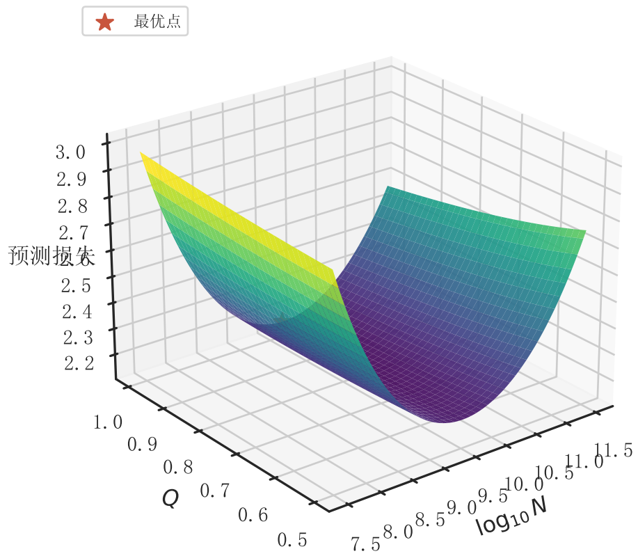
(N, Q) 目标曲面 ( C=1e22 , \ell=8192 )
