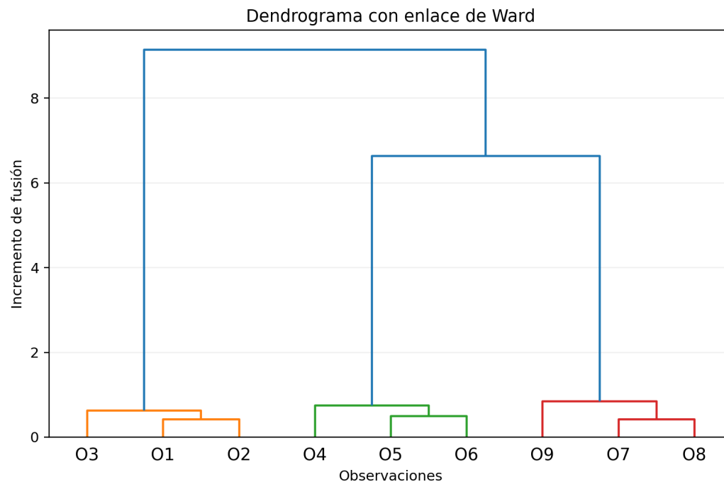
Figura 22.1: El dendrograma registra las fusiones y la altura a la que ocurren.
