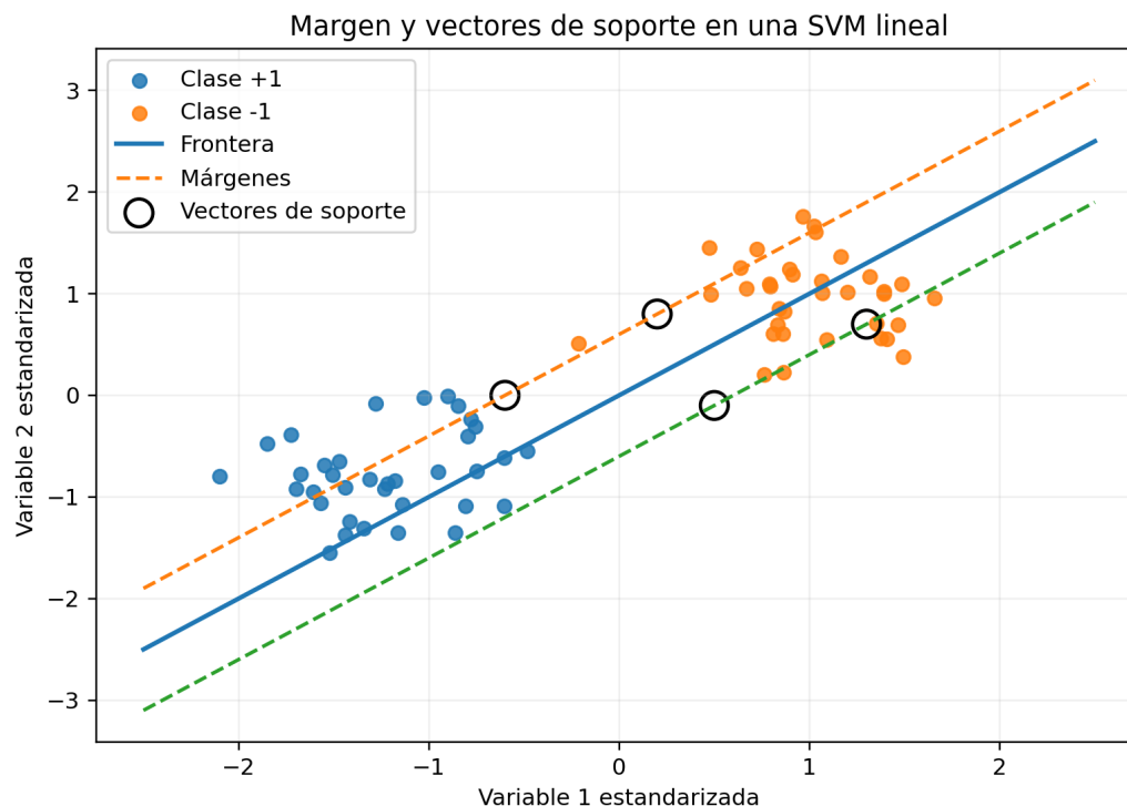
Figura 18.1: La SVM lineal busca una frontera con margen máximo y depende de los vectores de soporte.
