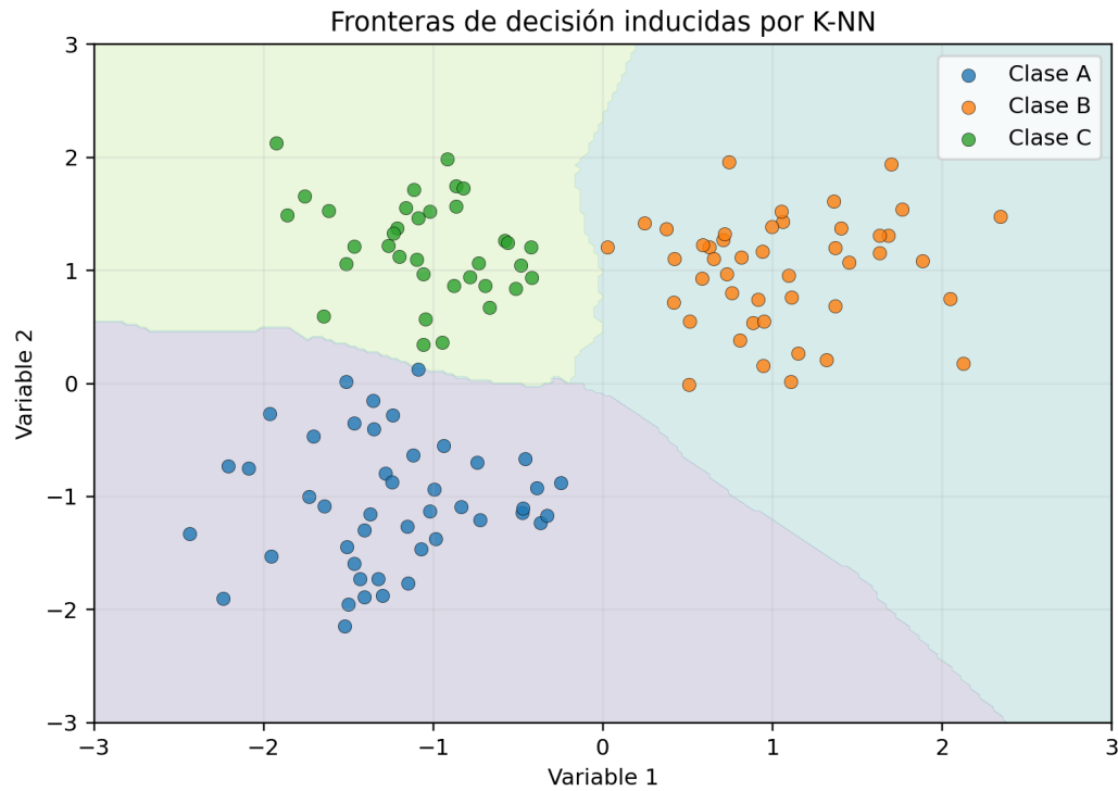
Figura 15.1: La elección de k y de la métrica determina regiones de decisión distintas.
