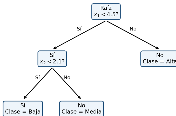
Esquema de un árbol de decisión
