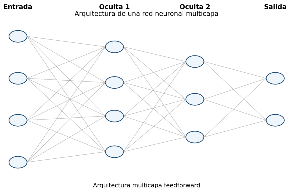
Figura 19.2: Una red neuronal multicapa transforma entradas en salidas mediante capas ocultas y activaciones no lineales.
