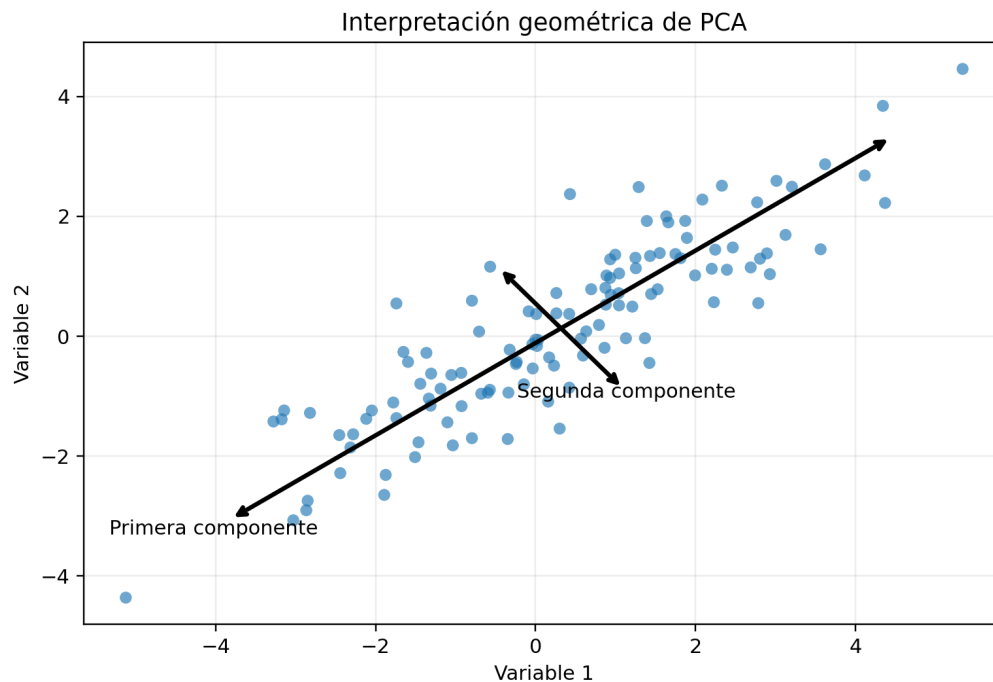
Figura 20.1: La primera componente sigue la dirección de máxima variabilidad; la segunda es ortogonal a ella.
