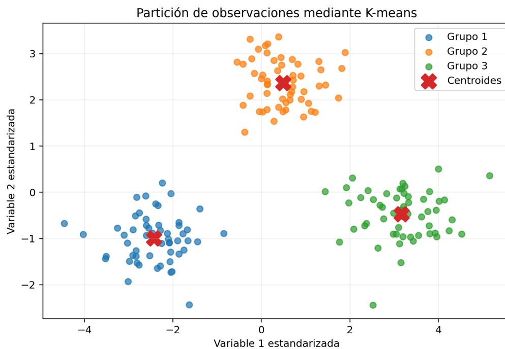
Figura 21.1: Los centroides resumen cada grupo y determinan regiones de asignación por proximidad.
