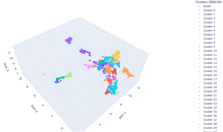
Figura 9: Projeção UMAP 3D com aplicação do algoritmo DBSCAN, evidenciando a fragmentação excessiva do supercluster.
