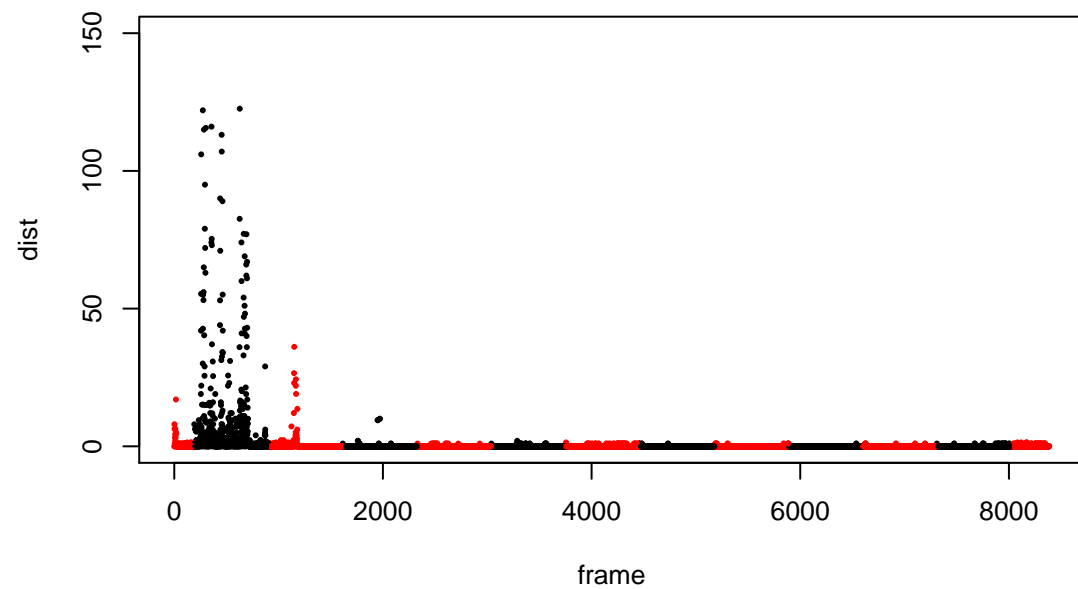
20140425-175349_0: ID: 5; sp: C_n
