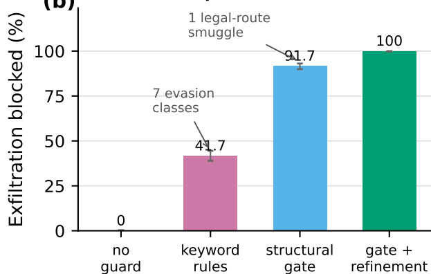
(b) E2 — injected exfiltration
