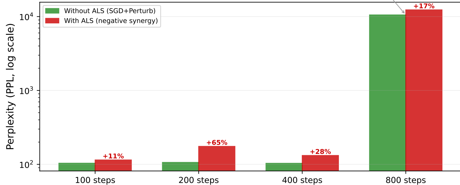
Figure 5: Low-Rank ALS Consistently Worsens Protocol C
