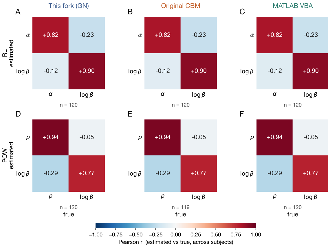
Figure 2 · Parameter recovery
