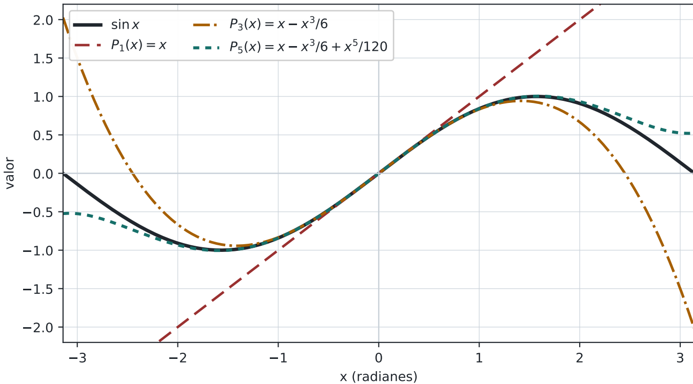
Aproximación local de \sin x en torno a 0
