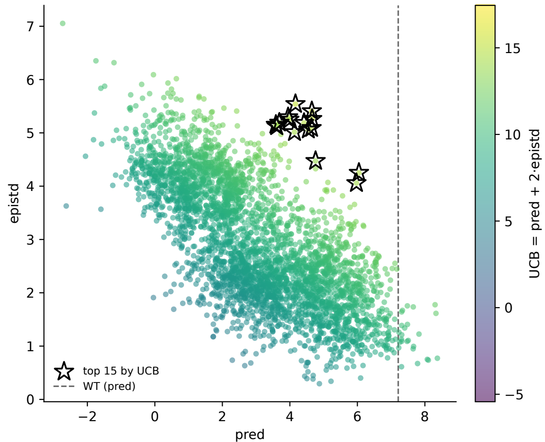
DPO 650M
