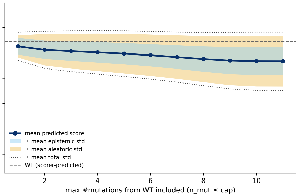
DPO 650M
