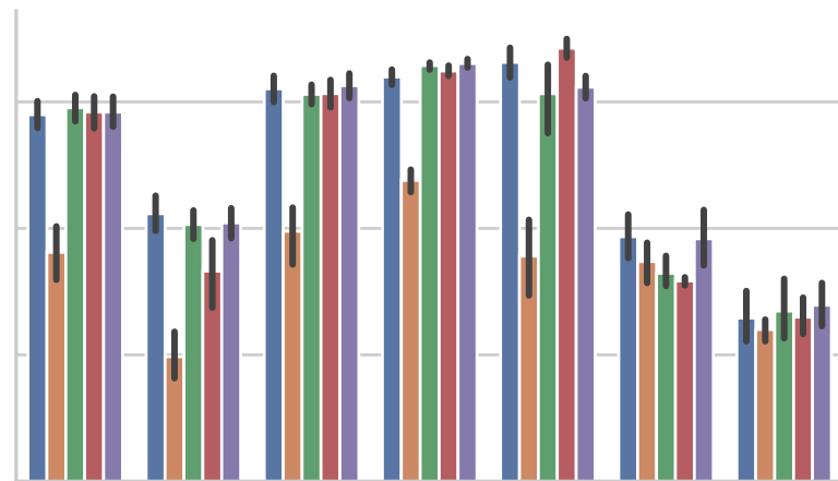
Precision
