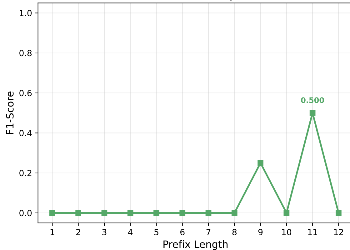
Recommendation System F1
