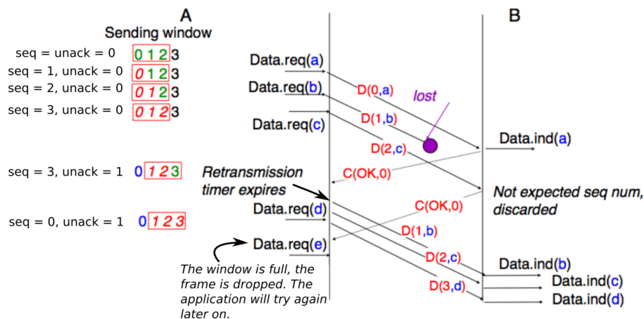
Figura 3.12: Go-back-n N=3, con errori [1]
