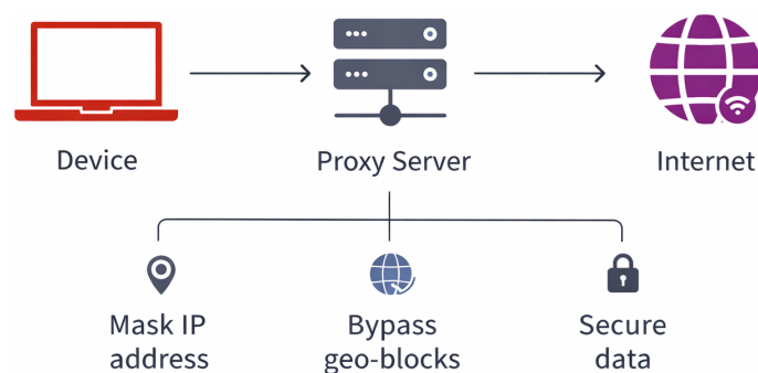
Figura 8.5: Server proxy
