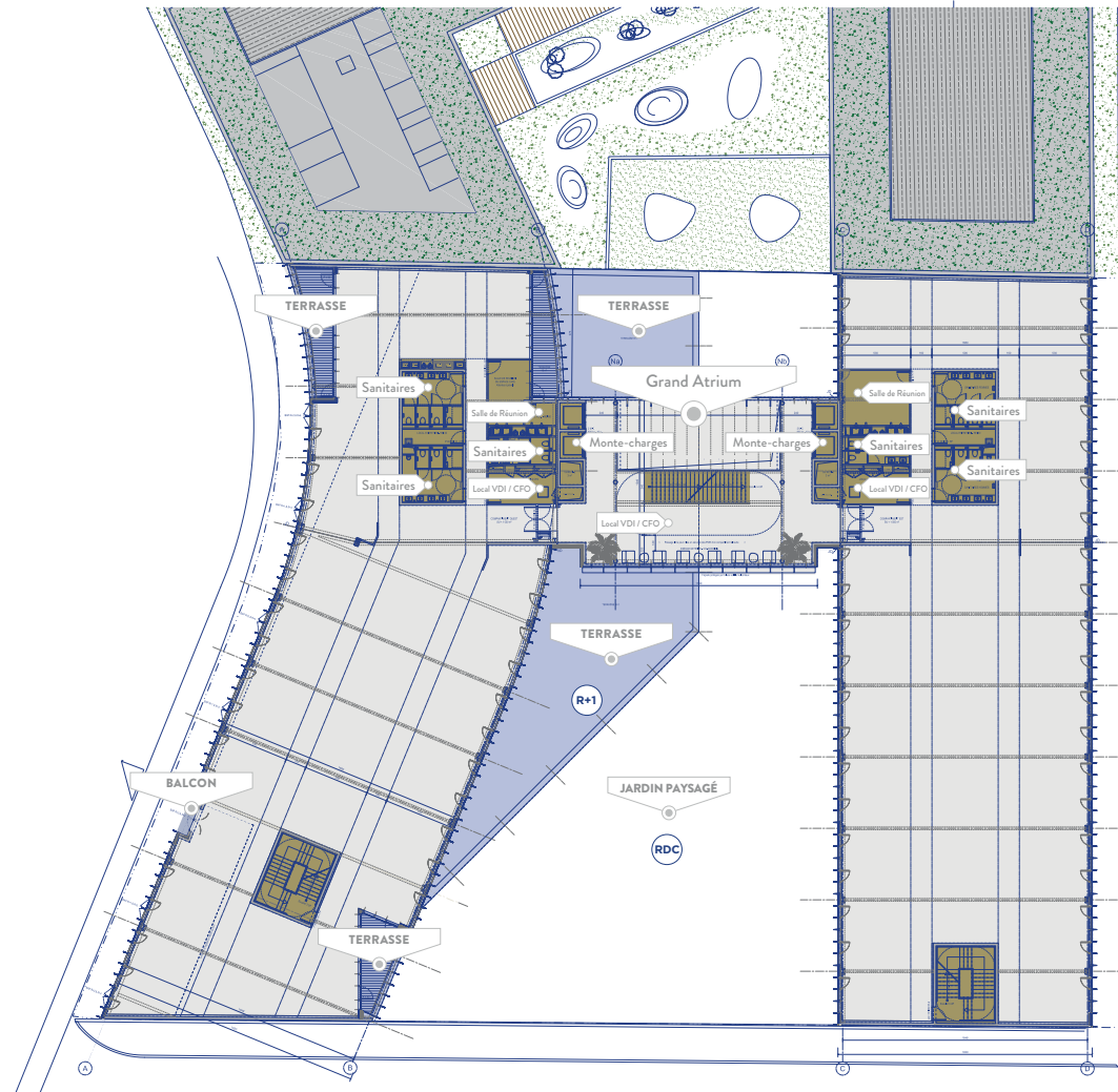
PLAN D'ÉTAGE COURANT : R+2
