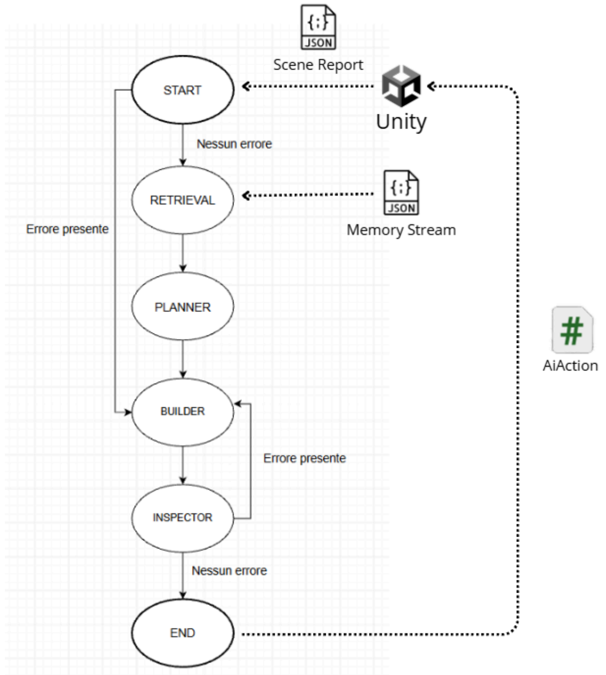
Figura 3.2: Panoramica del lato server di AmbraIA.
