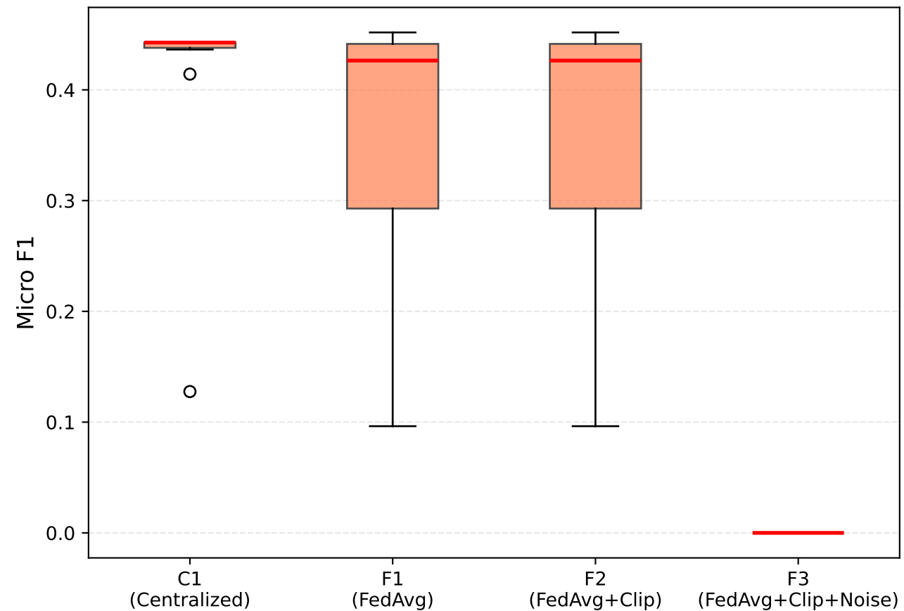
(b) Micro F1 Distribution (10 seeds)
