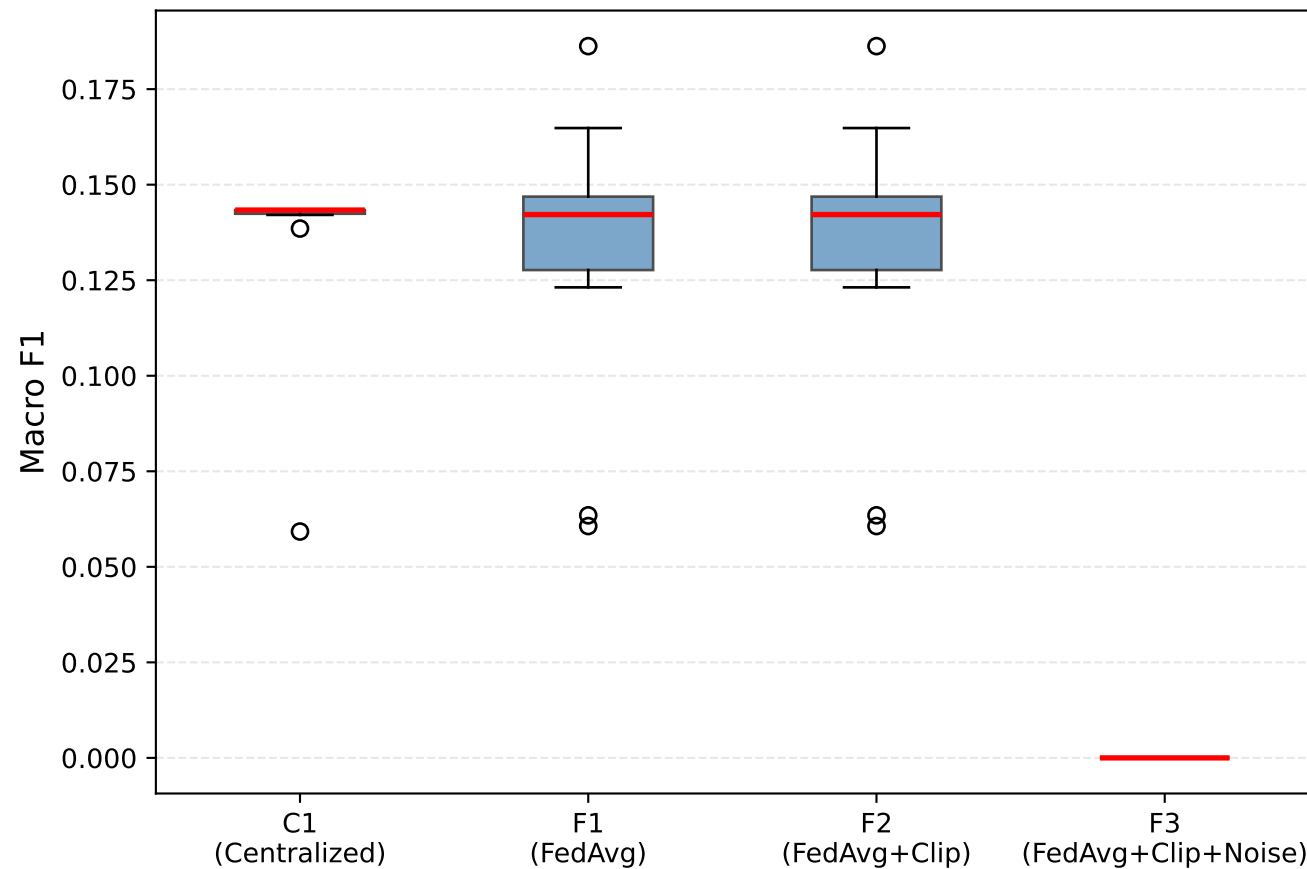
(a) Macro F1 Distribution (10 seeds)
