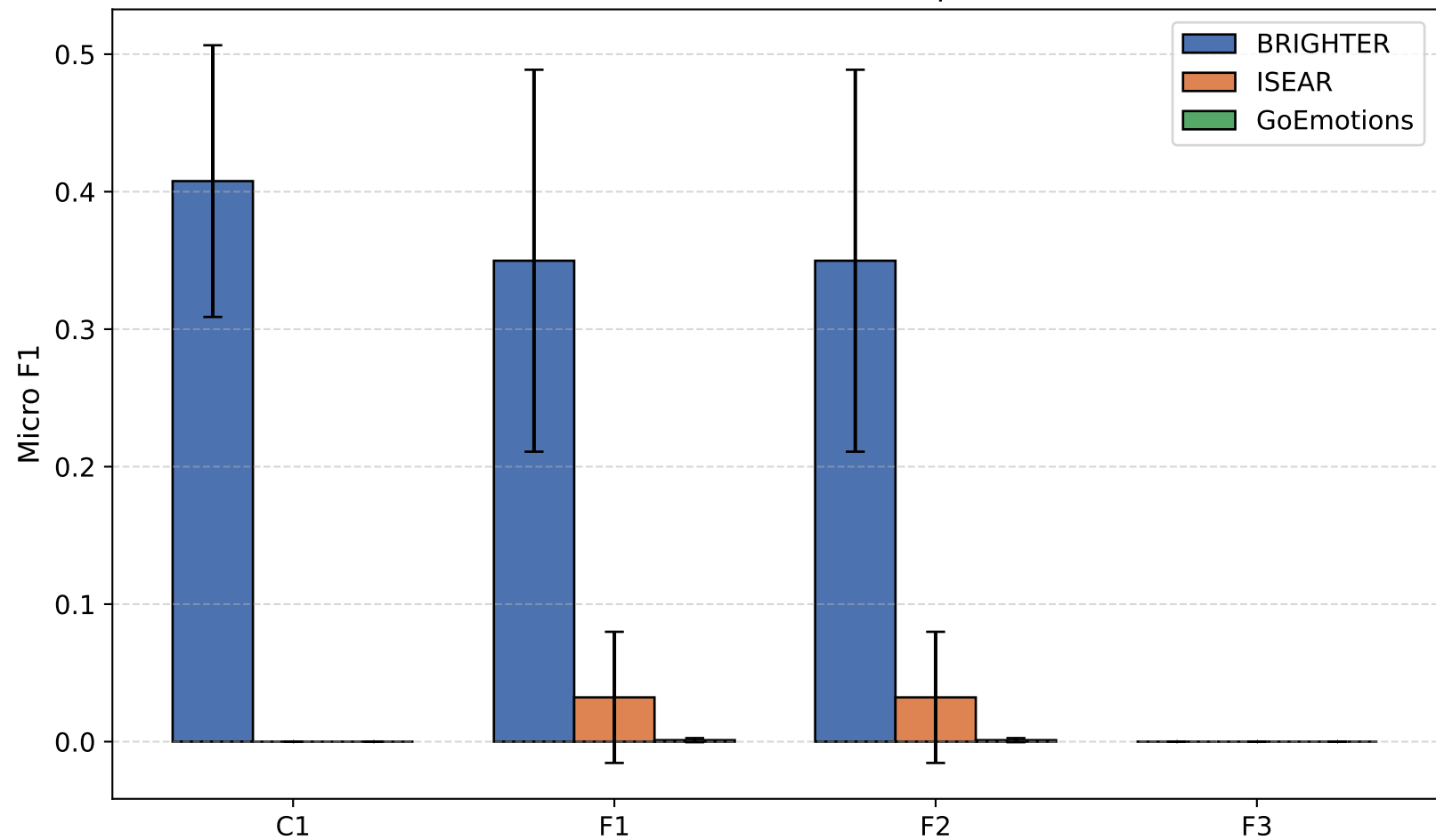
Cross-Dataset Micro F1 Comparison
