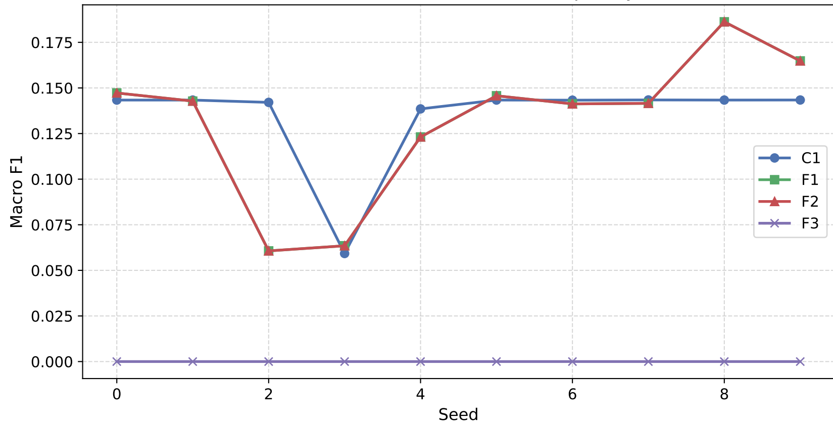
BRIGHTER: Per-Seed Macro F1 Trajectory
