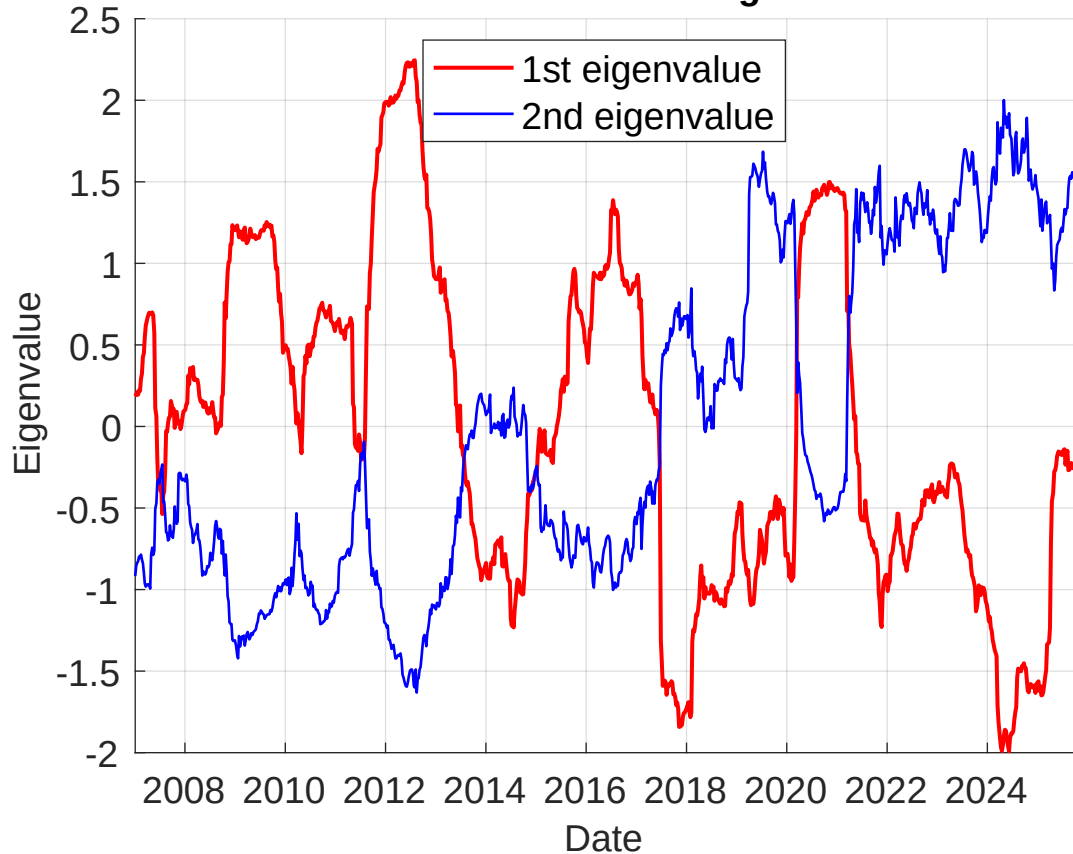
OMXS30: Standardized eigenvalues
