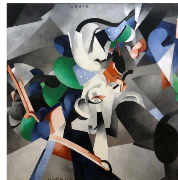
udnei*.onnx
