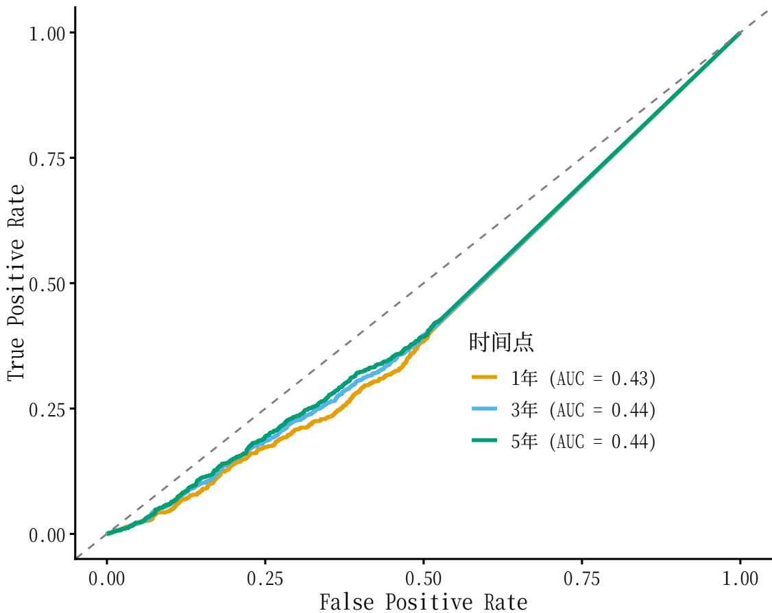
tsRNA_Asn_i_0144 的时间依赖ROC曲线
