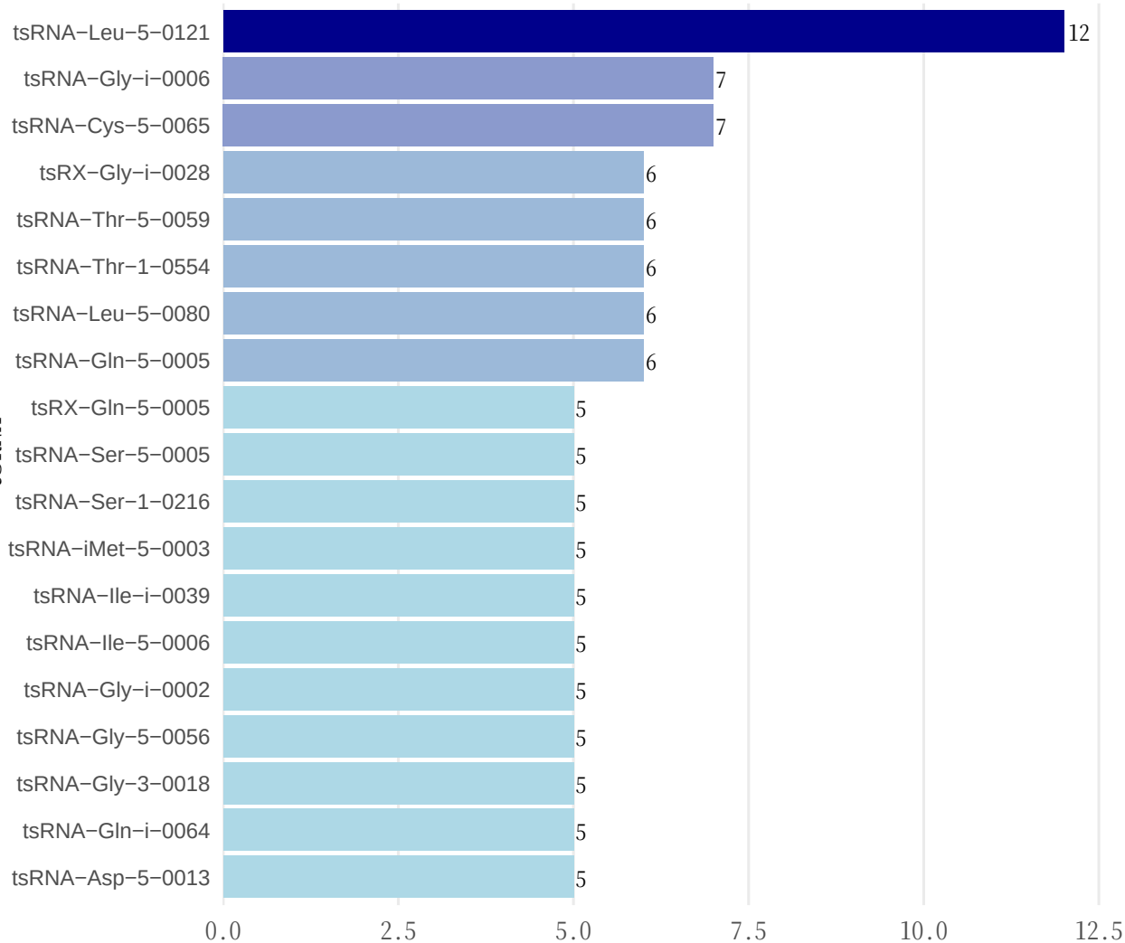
跨癌种高频tsRNA频次分布 (频次 \geq 5 )
