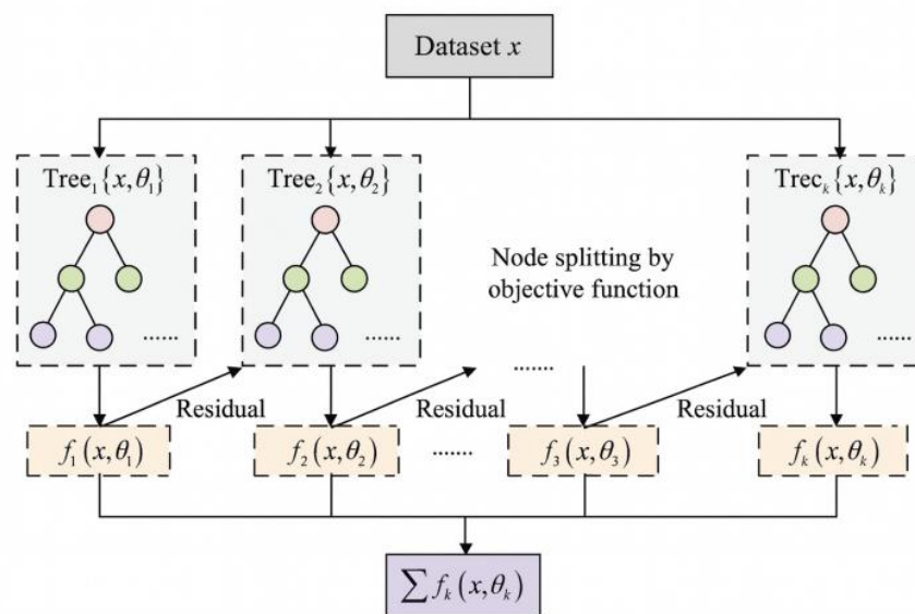
Hình 3.5 Boosting Algorithms
