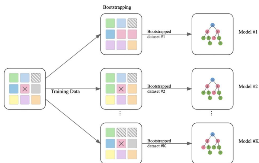
Hình 3.4 Bagging Algorithms
