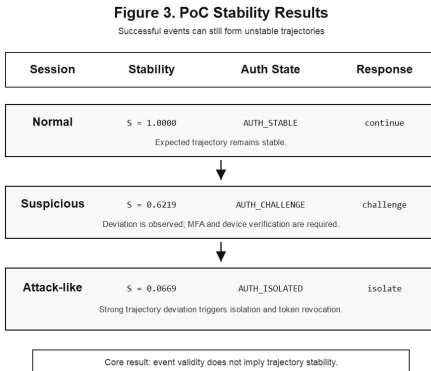
図 3: 正常・疑わしい・攻撃的セッションに対するPoC Stability結果。
