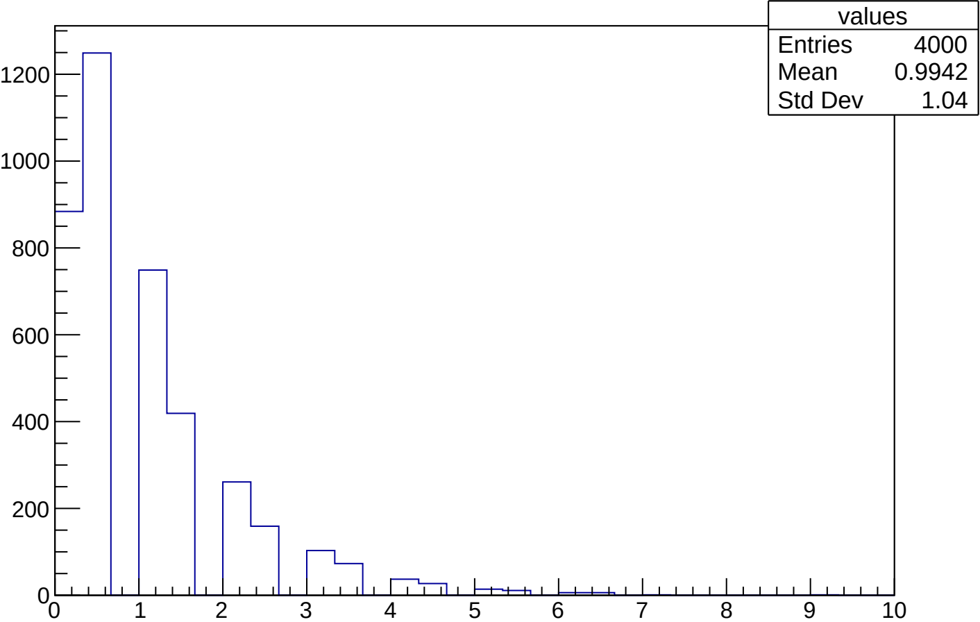
exponential_NO_round_2_values
