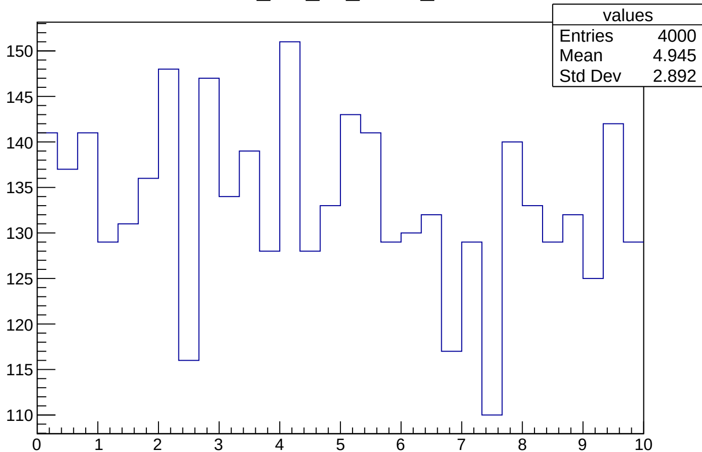
uniform_NO_no_round_values
