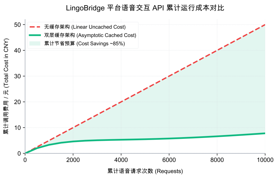
图 2.1 LingoBridge ASR/TTS 计费开销在双层缓存优化前后的走势对比
