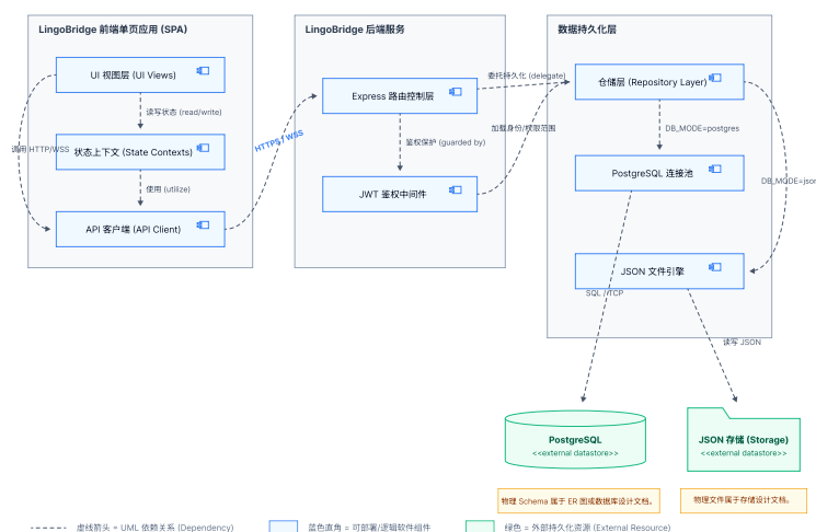
图 3.1 LingoBridge 系统核心组件与模块物理结构关系图
