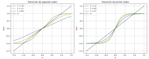
Figura 3: Representación gráfica de la ecuación de autocoherencia para transiciones de segundo y primer orden.
