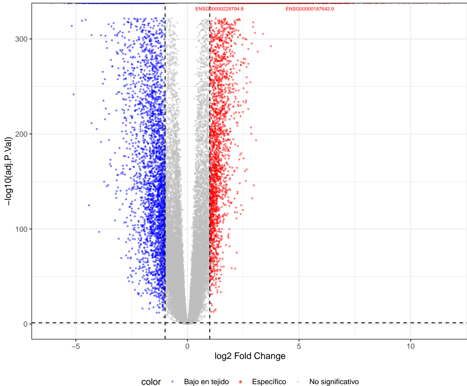
Volcano plot: HEART vs Resto
